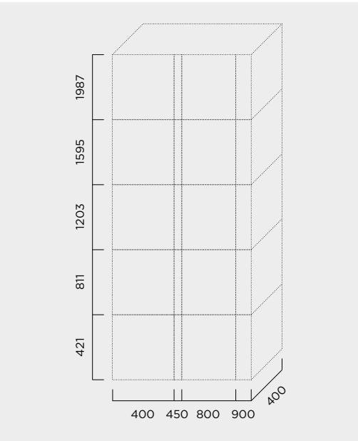
MIZO MODULGRÖSSEN IM ÜBERBLICK Angaben in mm
